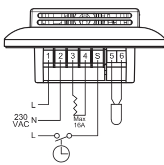
Подключение OTN2-1991
