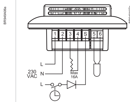
Подключение OTD2-1999 (режим защиты от замерзания)
